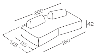
GRECD200
