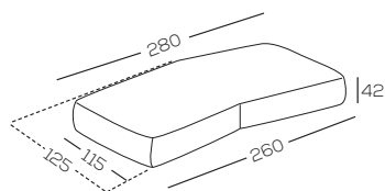
GRECB280
