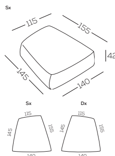
GRECB155 Dx/Sx
